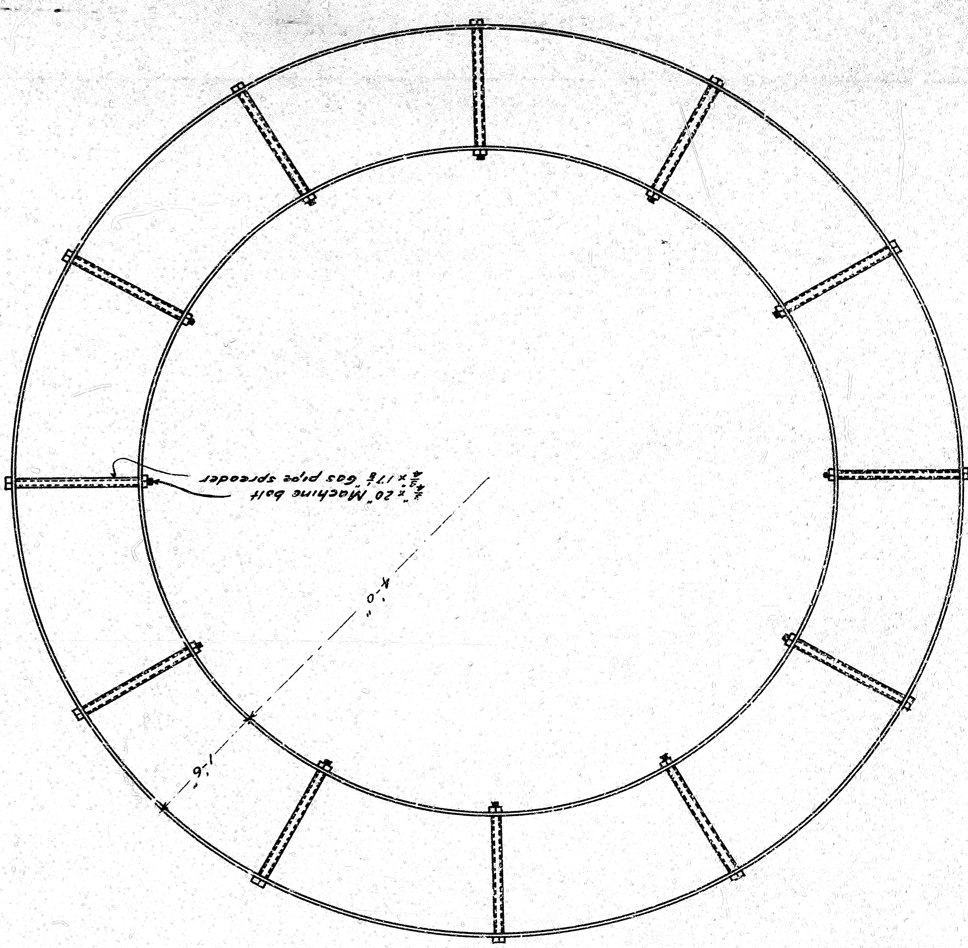
-PLAN-OF-SHOE-
